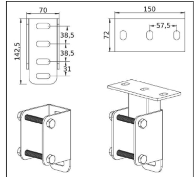
МОНТАЖНИ КОНЗОЛИ
